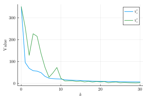
(c) Eigenvalues
